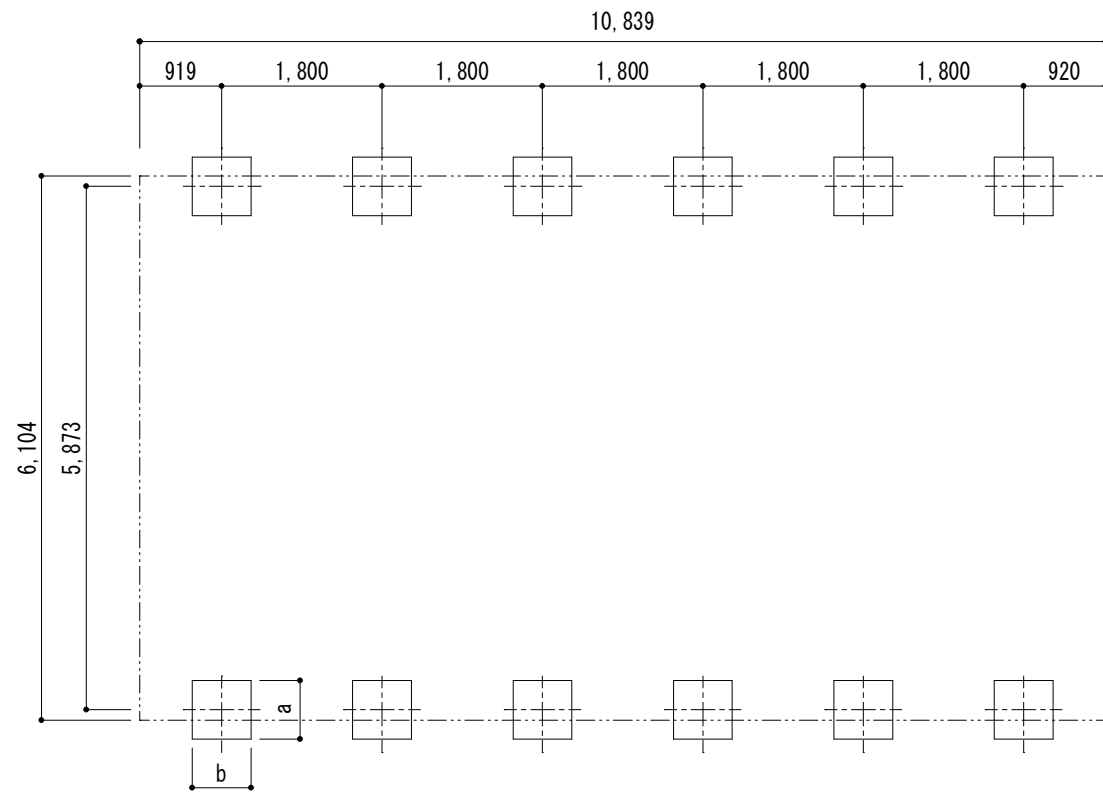
■基礎配置図
